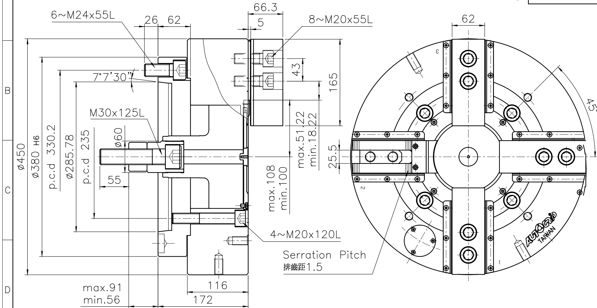
中實立車四爪夾頭
